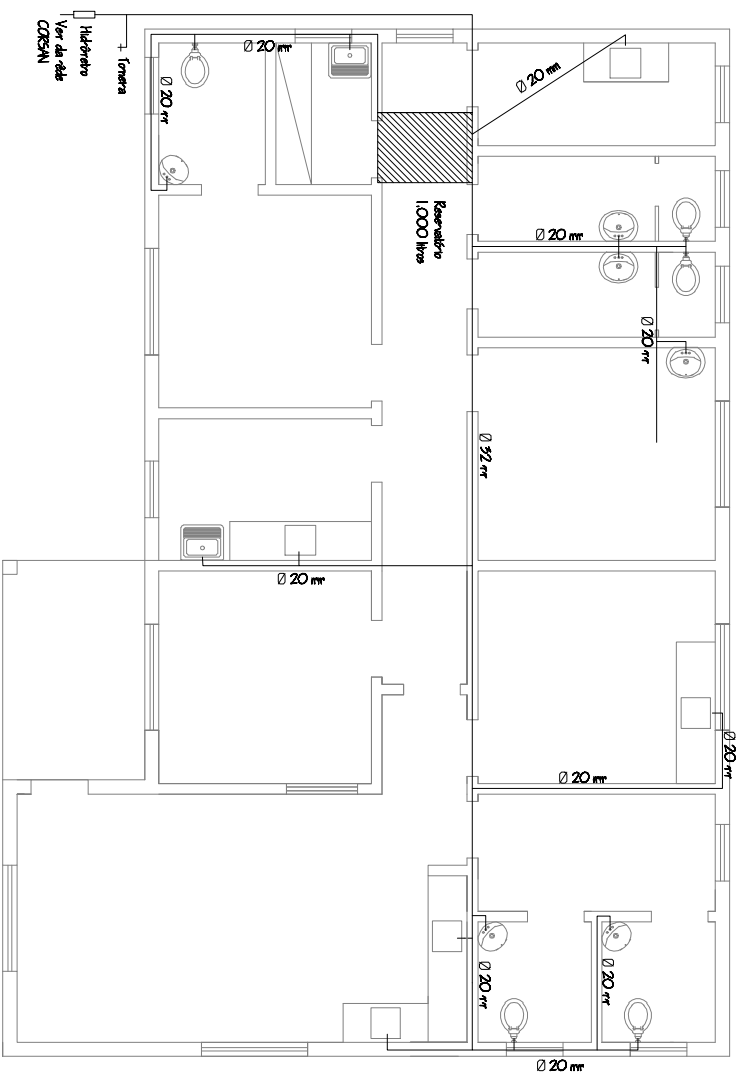
Projeto Hidráulico
