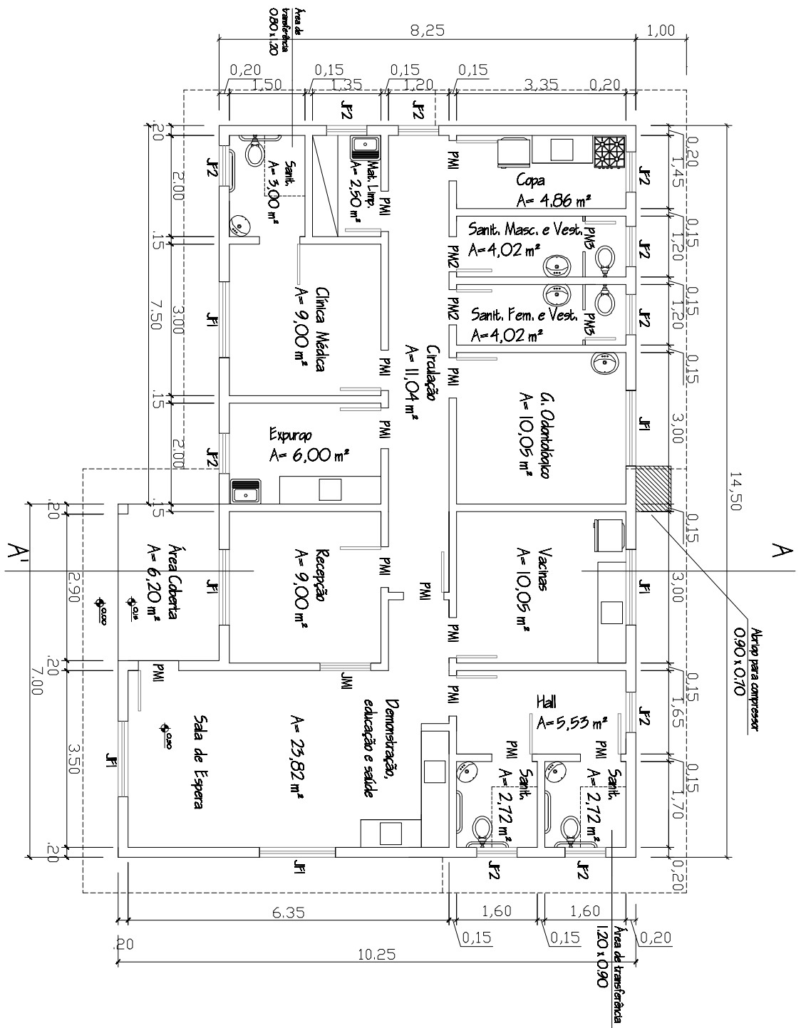
Planta Baixa
